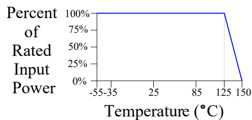
额定功率温度特性曲线
